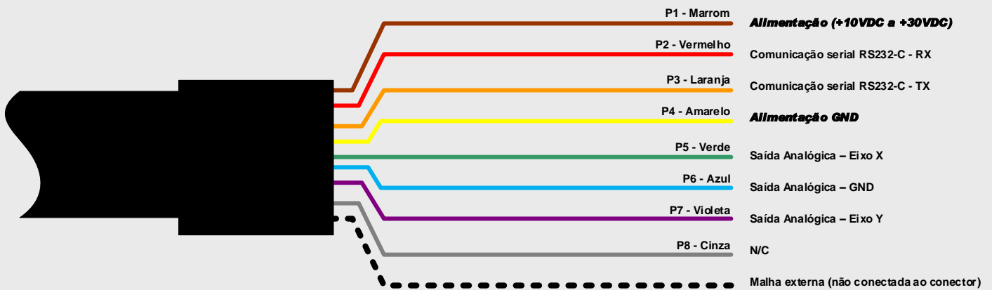
Esquema elétrico do cabo de conexão CA20 - REV-B (com conector Binder Série 713, COD 99-0486-12-08 montado com cabeamento)
