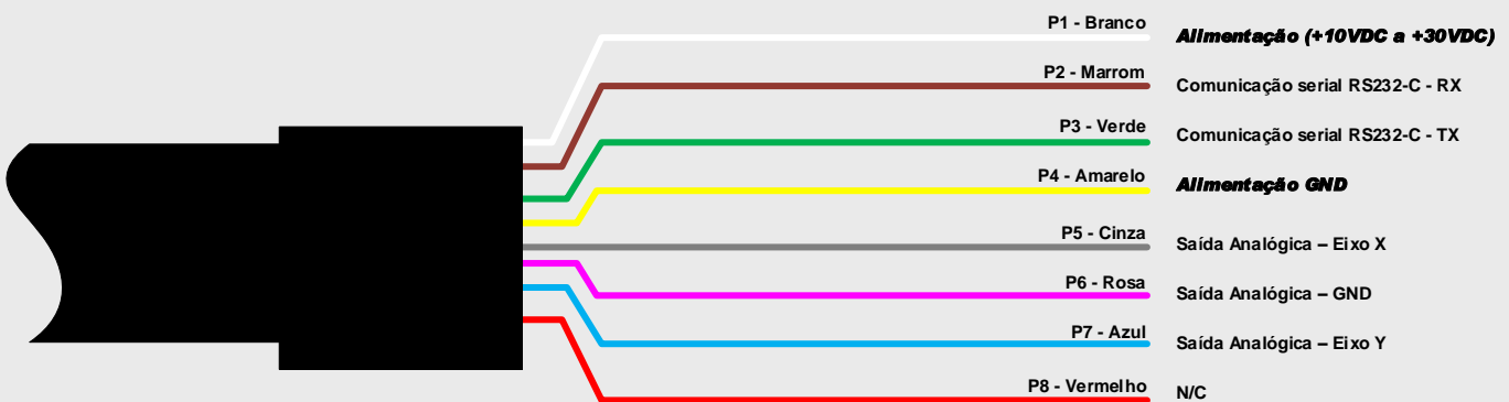
Esquema elétrico do cabo de conexão CA20 - REV-C (cabo Binder Série 763, COD 77-3430-0000-50708-XXX com conector sobre-injetado ao cabeamento)
