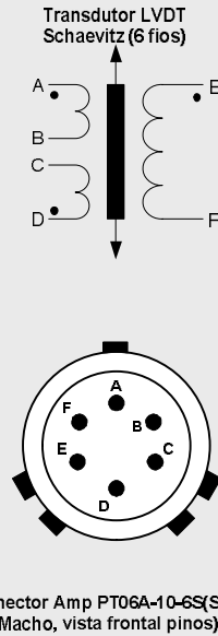
Esquema elétrico de ligação dos enrolamentos ao conector traseiro do transdutor (conector integrado ao corpo)
