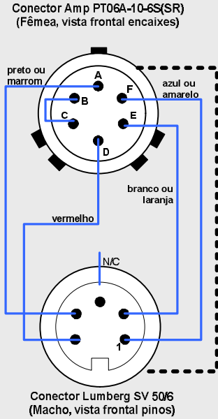
Esquema elétrico do cabo de conexão dos transdutores HCA e GCA
