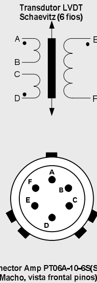
Esquema elétrico de ligação dos enrolamento ao conector traseiro do transdutor (conector integrado ao corpo)
