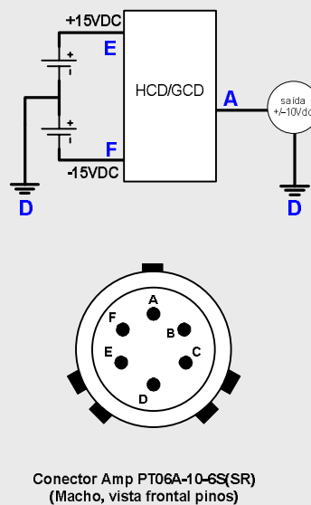
Esquema elétrico de ligação dos enrolamento ao conector traseiro do transdutor (conector integrado ao corpo)
